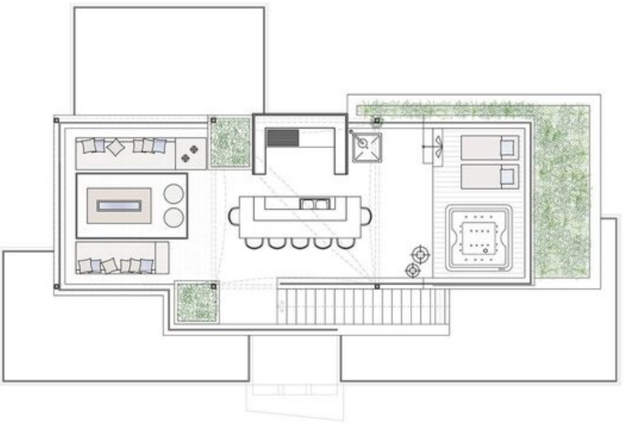
PLANTA CUBERTA
