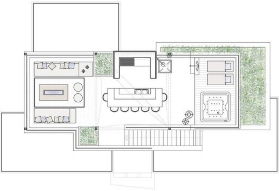
PLANTA CUBERTA
